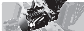
Framed central differential triangle bracket Support de triangle différentiel central encadré Gehäufte zentrale differenzielle Dreieckshalterung Soporte triangular diferencial central enmarcado 框式中央差速三角支架
